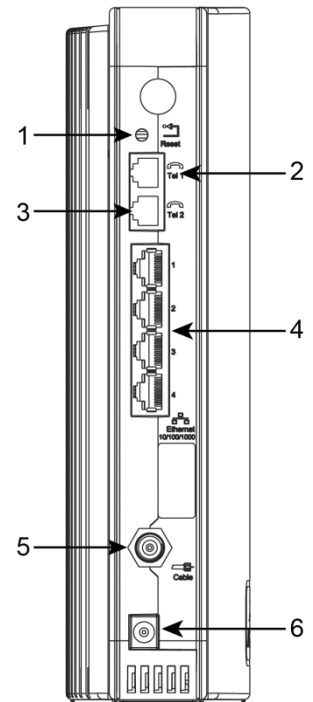
Kuva 1, liitännät
